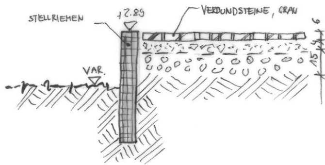
TERRAIN, HÖHENABSATZ
